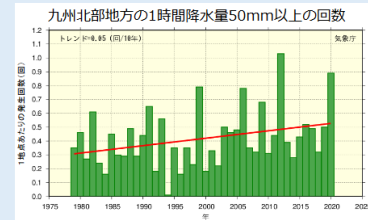
緑の棒：各年の1時間降水量50mm以上の回数 赤の直線：この期間の長期変化傾向
