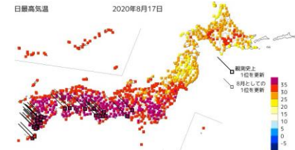
2020年8月17日の 日最高気温 (出典：気象庁)
