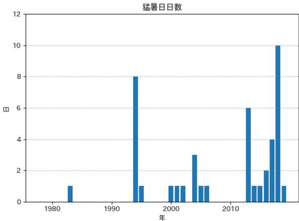
図 11 猛暑日数の推移 (防府市)
