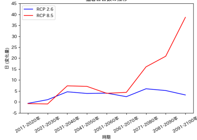
図 27 猛暑日の推移予測 (防府市)
