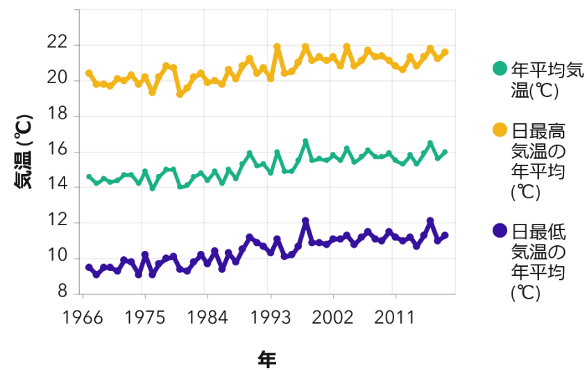
気温の推移（年別値）（山口市）
