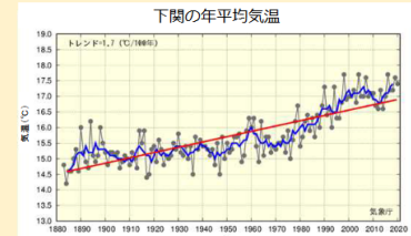
黒の細線：年平均気温 青の太線：気温の5年移動平均 赤の直線：この期間の長期変化傾向 ※地球温暖化に加え都市化や自然変動も含む
