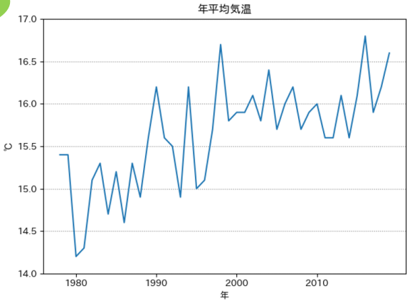
図 7 年平均気温の推移 (防府市)
