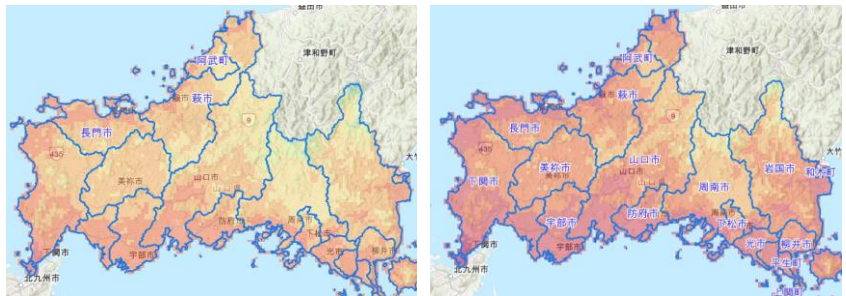
2°C上昇シナリオ
