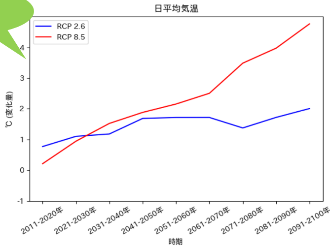
図 18 日平均気温の推移予測 (防府市)
