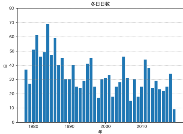
図 12 冬日数の推移 (防府市)
