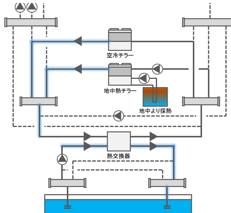
蓄熱フロー(夜間蓄熱時)
