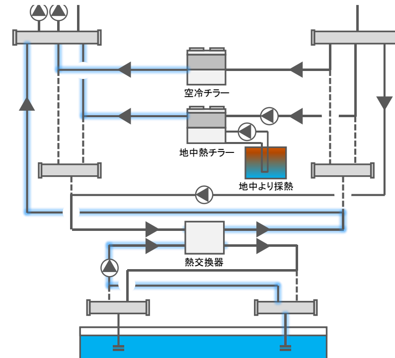
蓄熱フロー(昼間放熱時)
