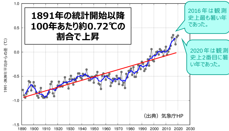
世界の年平均気温の変化（基準値は1991-2020の30年平均值）
