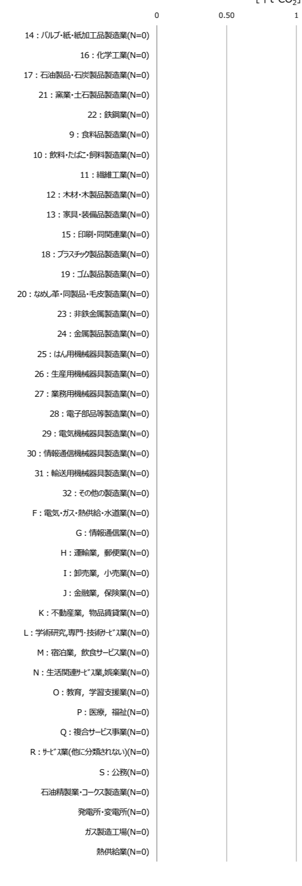
区域のエネルギー起源CO2排出量 [kt-CO2]
