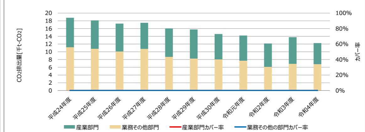
区域のエネルギー起源CO2排出量 [kt-CO2]
