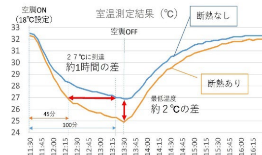
断熱改修の試験施工による 省エネ効果の測定結果（清和小学校）
