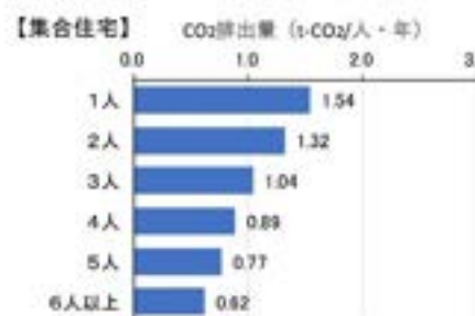
H28 年家庭からの CO2 の推計に係る実地調査 (環境省)
