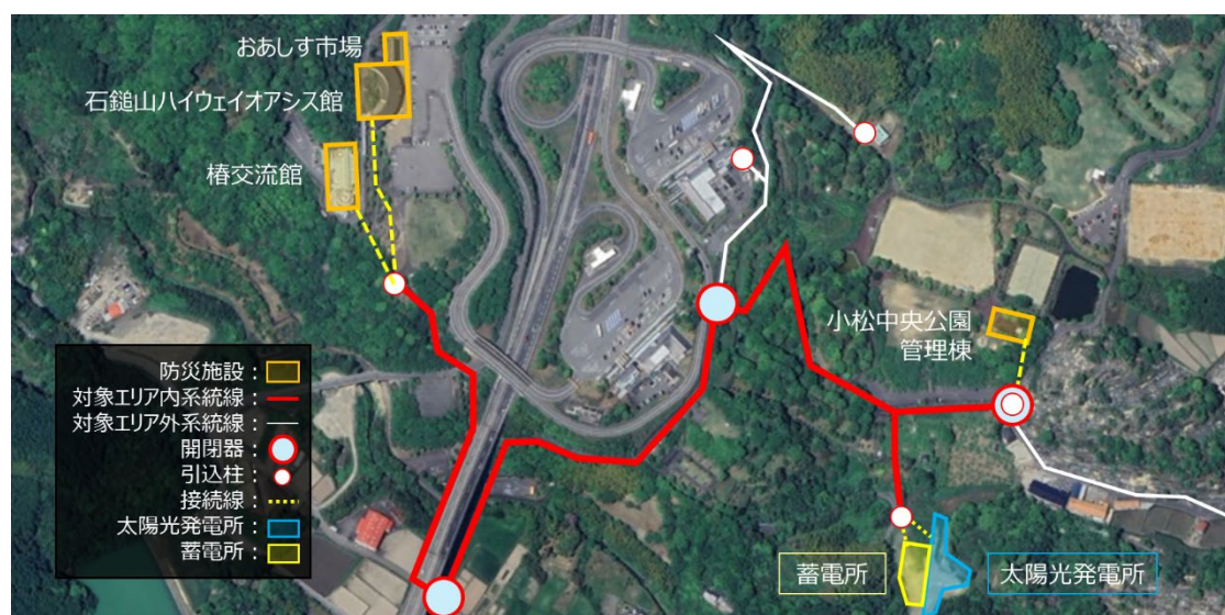
系統線マイクログリッド構築エリア及び設備配置図
